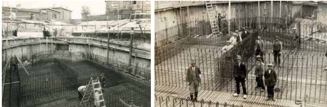
Rioolgemaal slachthuis-terrein Den Haag in uitvoering. Zichtbaar zijn de gewapend-beton-constructies van de funderingen. Op de linker foto staat Jan den Ouden achterin, op de rechter Arie, bij de trap. Beiden met gleufoed, 1925.
