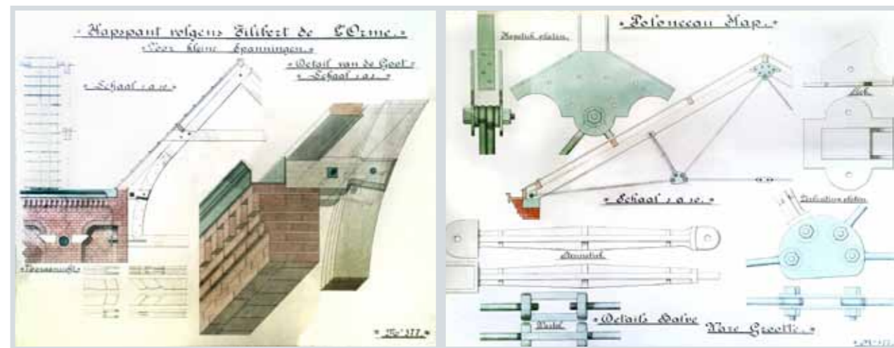
Links: Kapspant volgens Filibert de l'Orme. Jan maakte deze tekening voor het vak Bouwkundig- en Vaktekenen voor timmerlieden op het eindexamen van de avondschool voor ambachtslieden, 1905. Rechts: 'Polonceau Kap'. 10 De linker tekening benadrukt het architectonisch-esthetische aspect van een kapconstructie, terwijl de rechter tekening de techniek van een dakconstructie laat zien.
